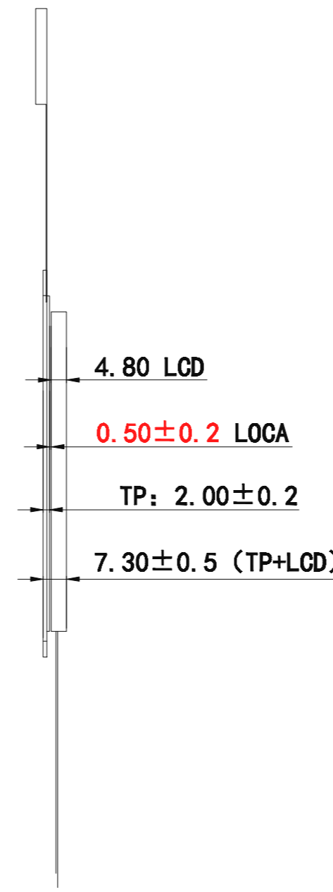
侧视图
