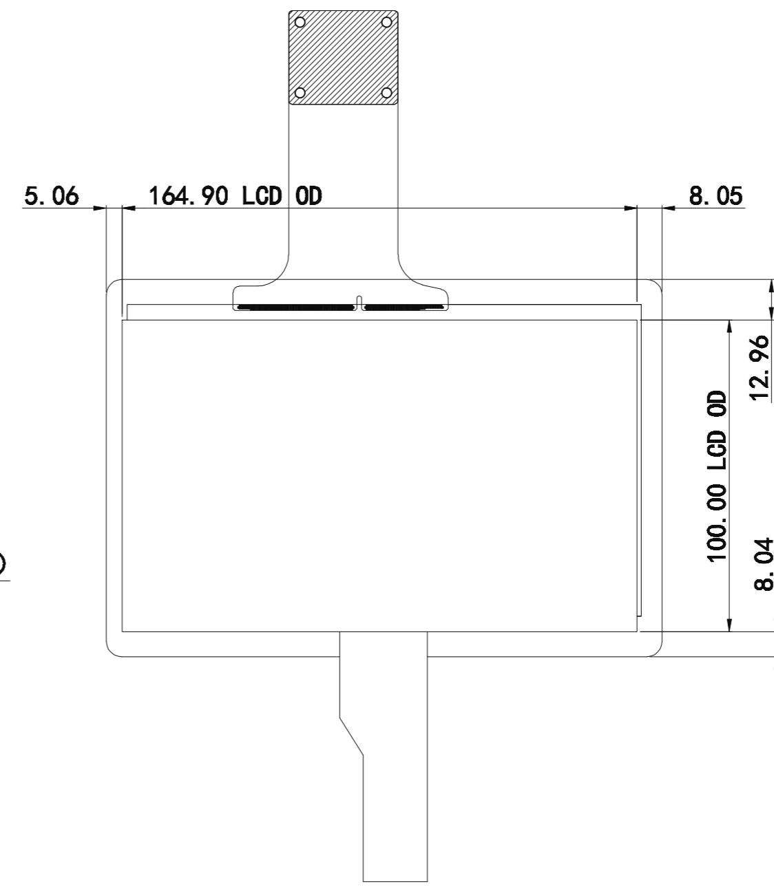
背视图
