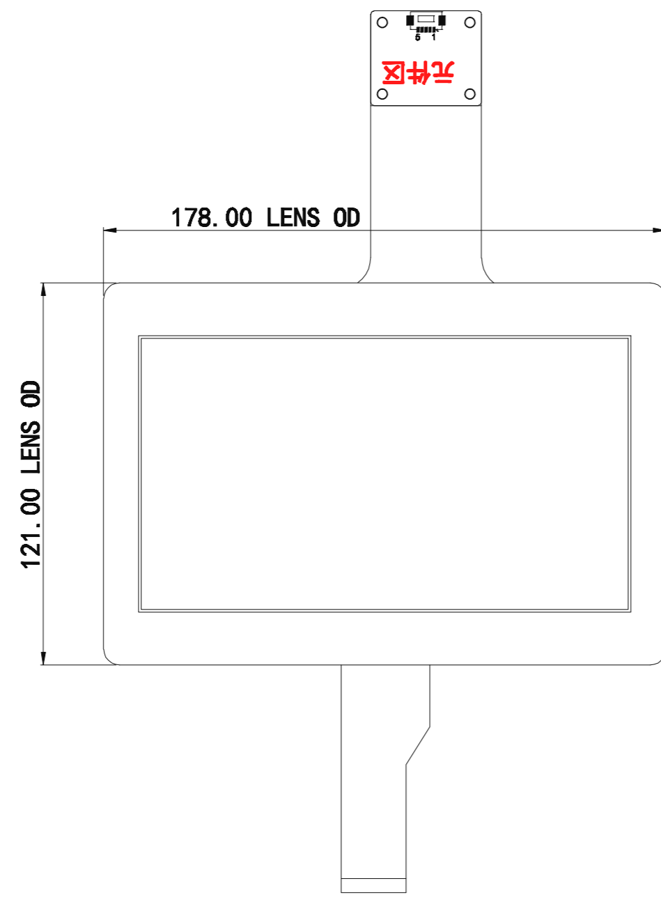
正视图
